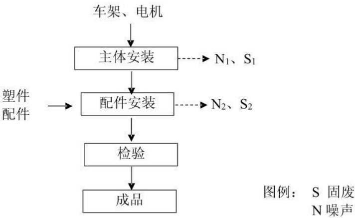
图 2-32 自行车组装生产工艺图
