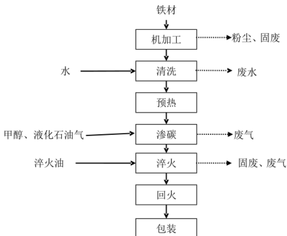
图 2-33 自行车配件生产工艺及产污环节
