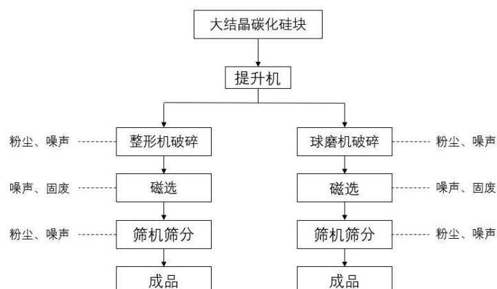
图 2-34 碳化硅微粉制造生产工艺图
