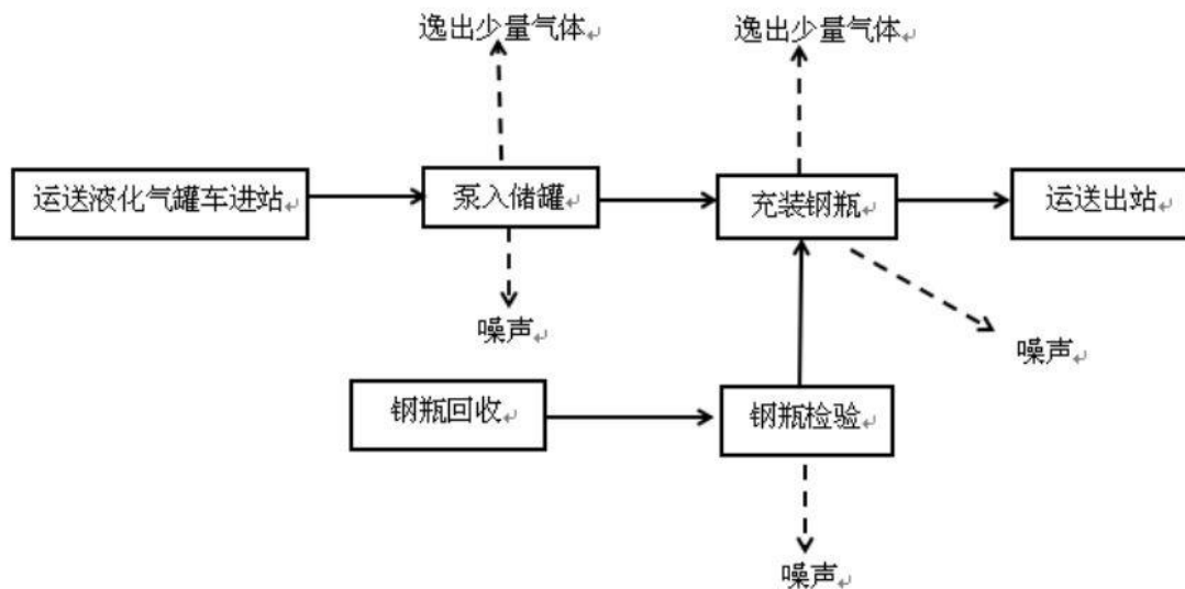
图 2-36 燃气经营工艺图
