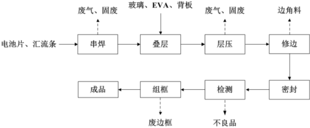
图 2-35 光伏设备生产工艺及产污环节
